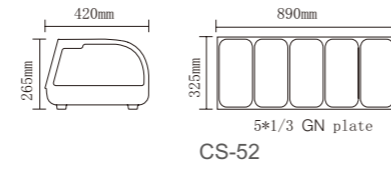
CS-52
