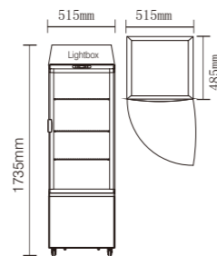
CL-218 (Lightbox)
