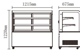
CW-370R
