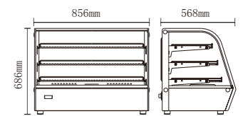
HW-160
