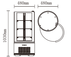
CL-100
