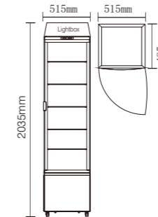
CL-288 (Lightbox)
