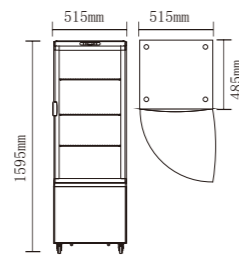
CL-218
