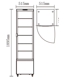
CL-288
