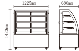
CW-371R
