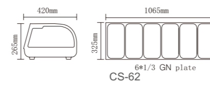
CS-62
