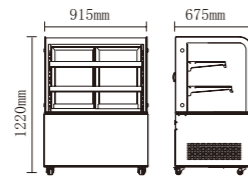
CW-270R
