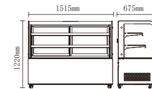
CW-470R
