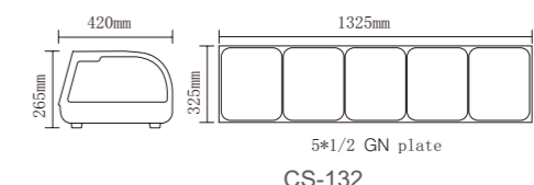
CS-132
