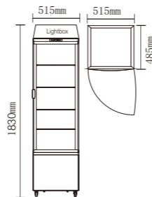
CL-238 (Lightbox)
