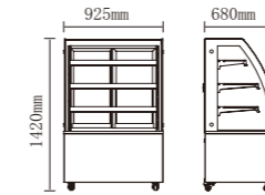
CW-271R
