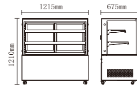
CW-370
